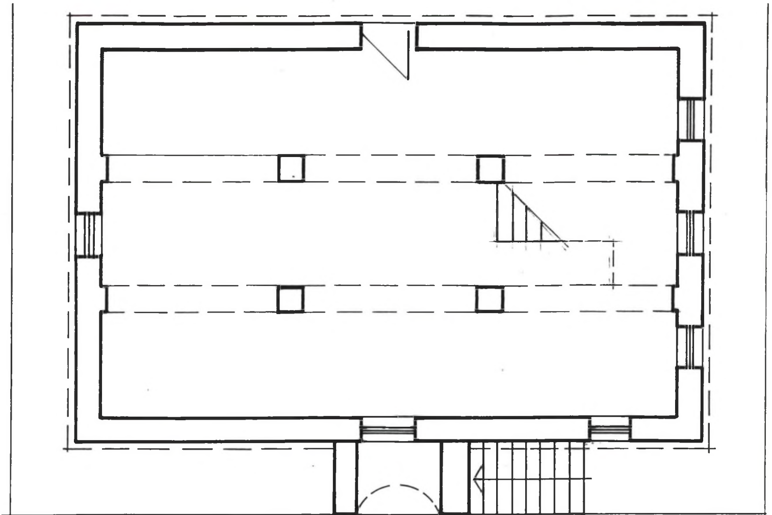
ΚΑΤΟΨΗ ΙΣΟΓΕΙΟΥ
